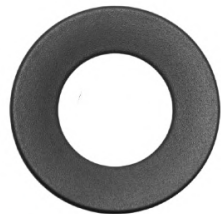
W11088240 SUP POW CAP EXTERIOR MATTE Tapa Quemador Exterior Xtreme, Diam. Ext 13.5 cm, Diam. Int. 6.5 cm
