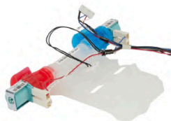
WPW10683603 IVVB ASSEMBLY, CLASSIC Válvula de Agua Con Termistor
